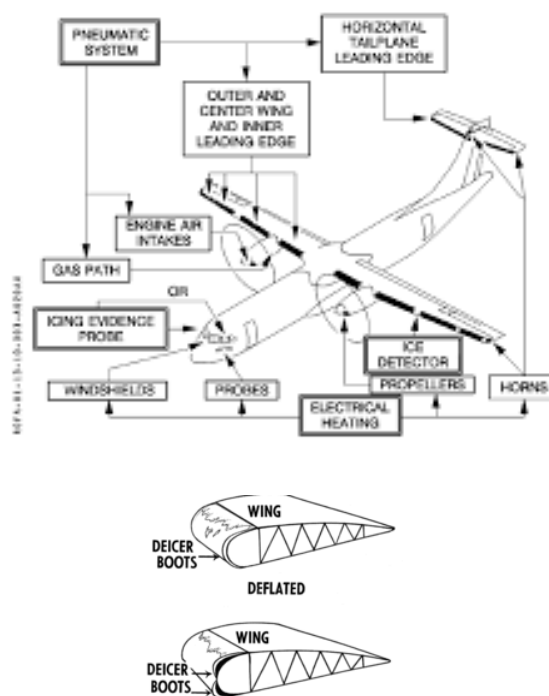
図. 3 ATR42 と ATR72 の防除氷装置
