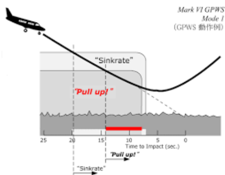
図.3 GPWS の警報
